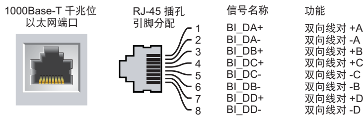
图 2 千兆位以太网端口引脚分配
